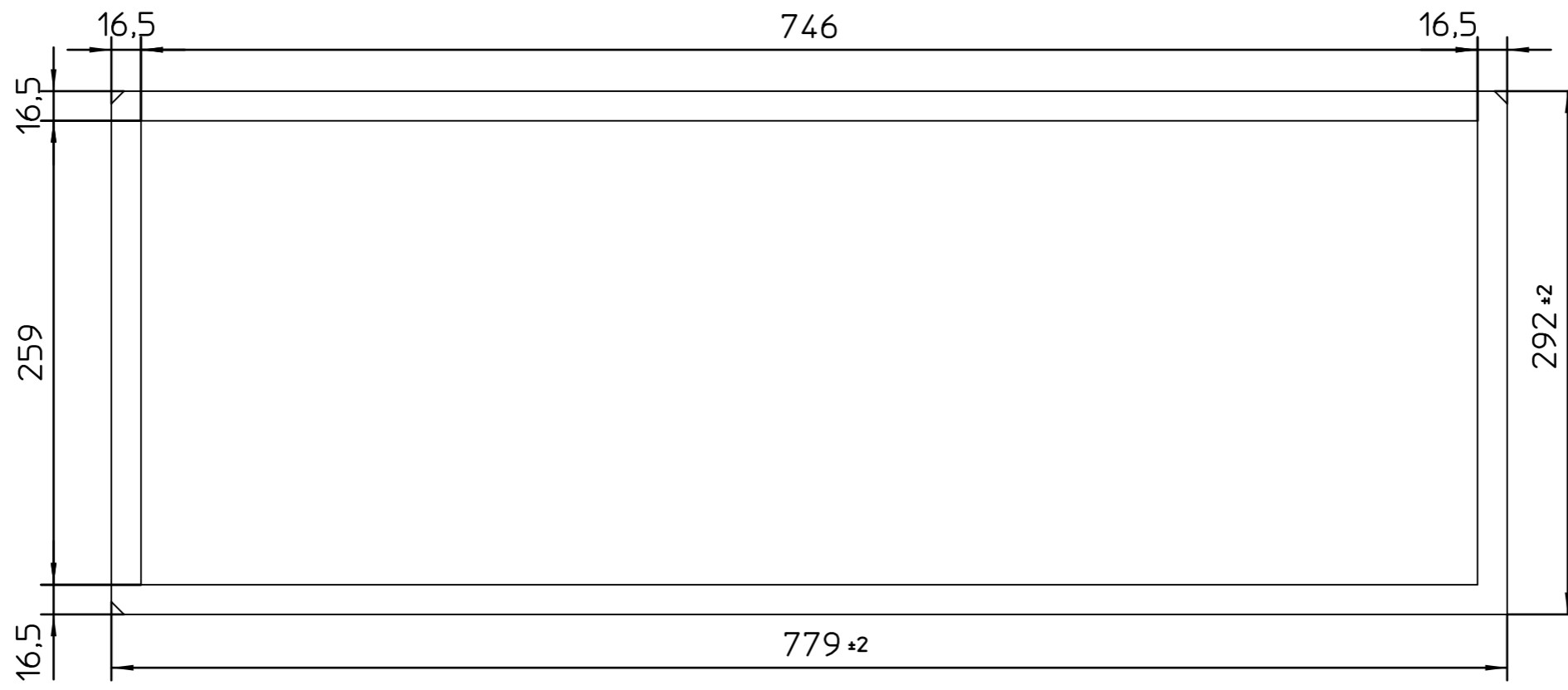
Vorderansicht 1 1:3.5
