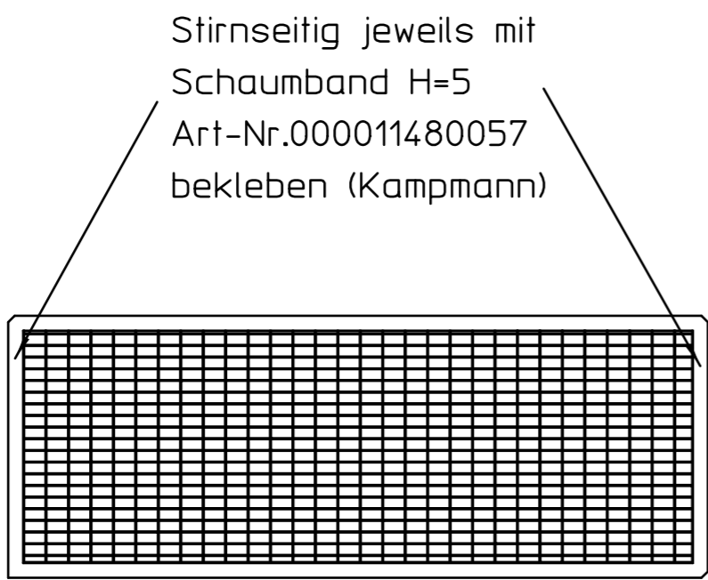
Rückansicht 1 1:7.5
